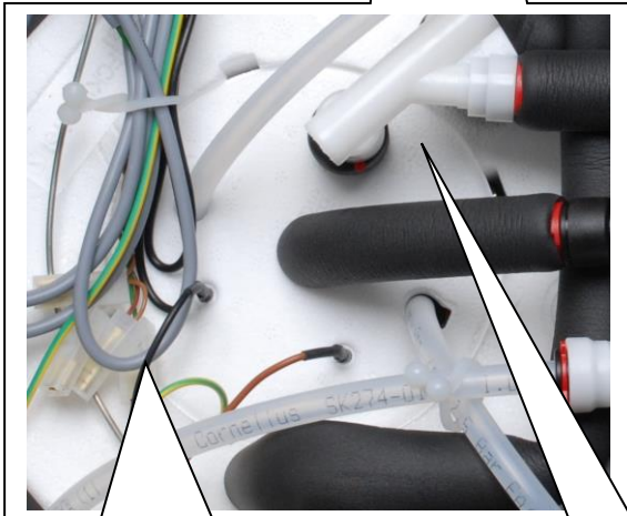
Niveausonde für Pumpensteuerung min = braun max = schwarz
